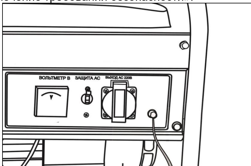
Рис. 4. Заземление
