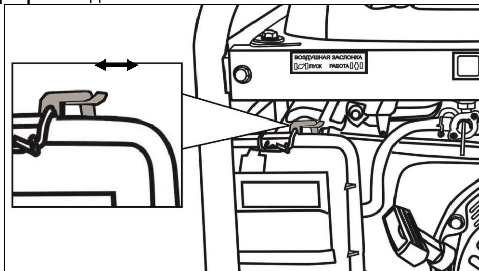
Рис. 8. Воздушная заслонка
