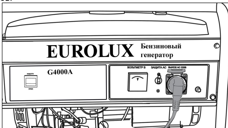
Рис. 11. Подключение потребителей
